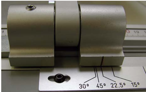
Abb. 12-5: Einstellung Anschlagklappe
