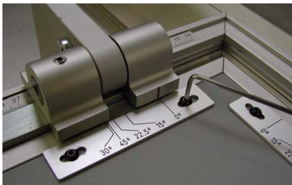
Abb. 12-3: Einstellung Längenausgleichskala
